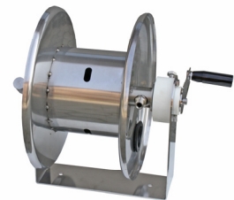
Arrotolatore Manuale Cod. 10420/X/BS (con tubo) Cod. 10400/X (senza tubo) (Sez. 51)
