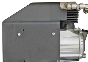
Compressore 0,75 Kw 400 V Trifase Cod. 86905
